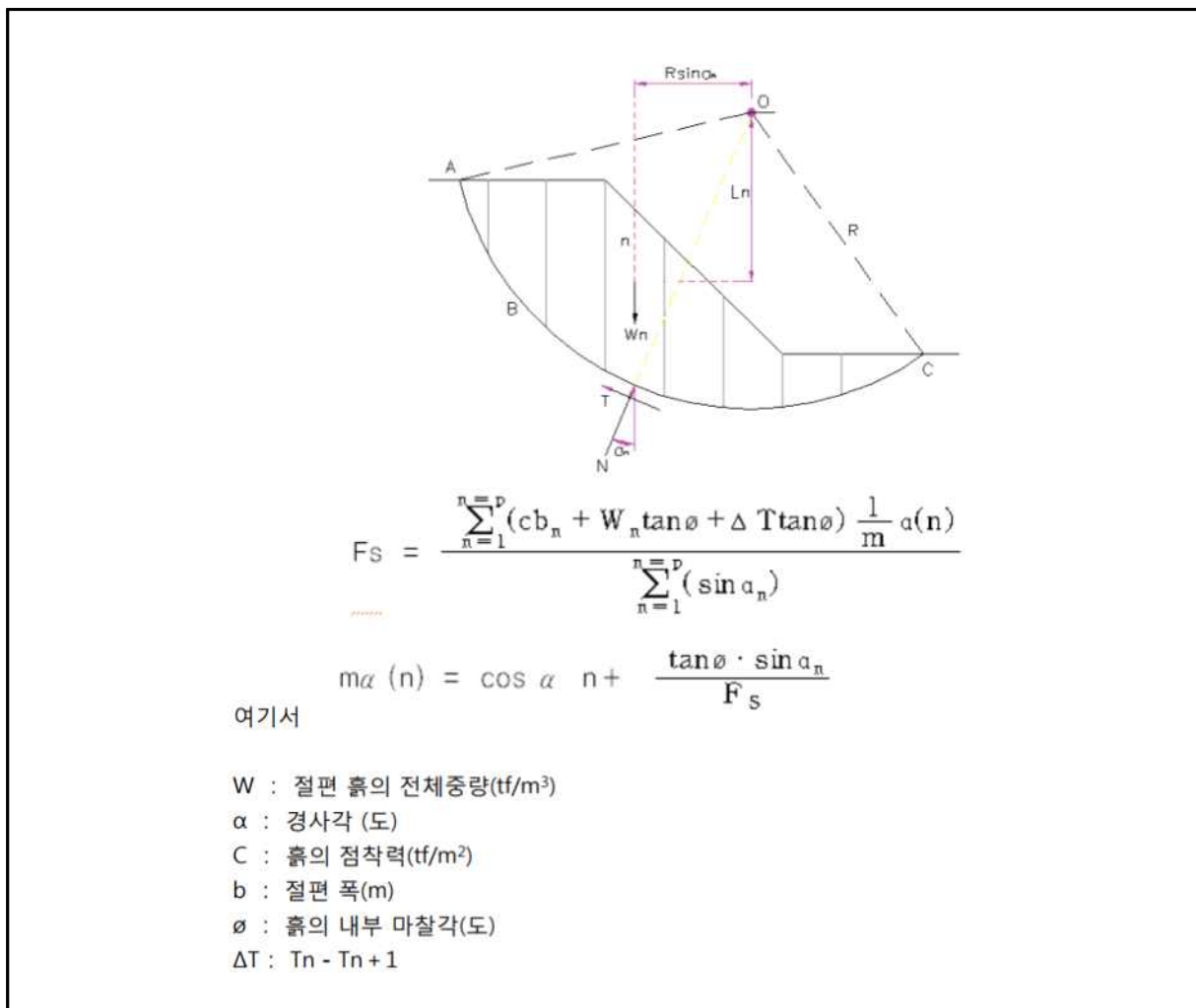
【그림 29.7】 Bishop의 안전을 계산식
